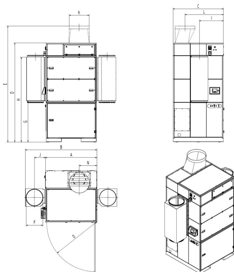
Fig. 62 : Fiche dimensionnelle 3475
